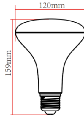
BR40 - 12W/17W
