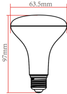
BR20 - 7W
