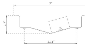
1 x 4 Troffer Retrofit
